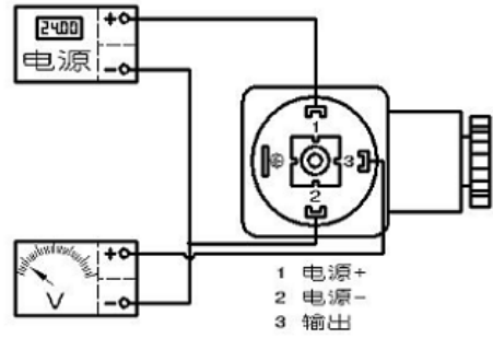
電壓信號
